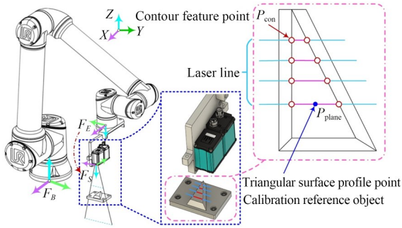
图1 机器人手眼标定参照物与特征提取示意图
